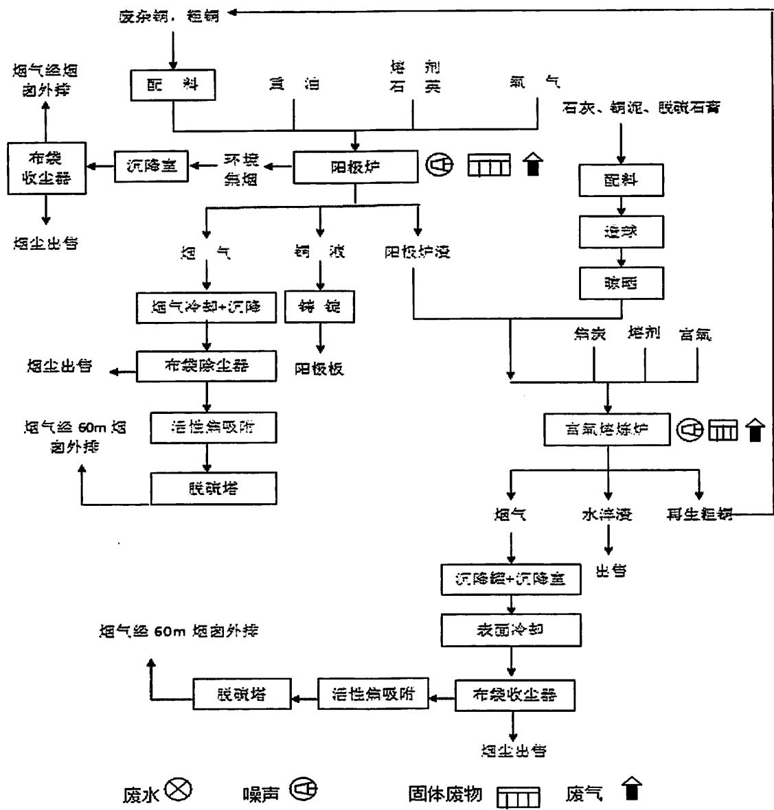
阳极铜生产线工艺流程图
