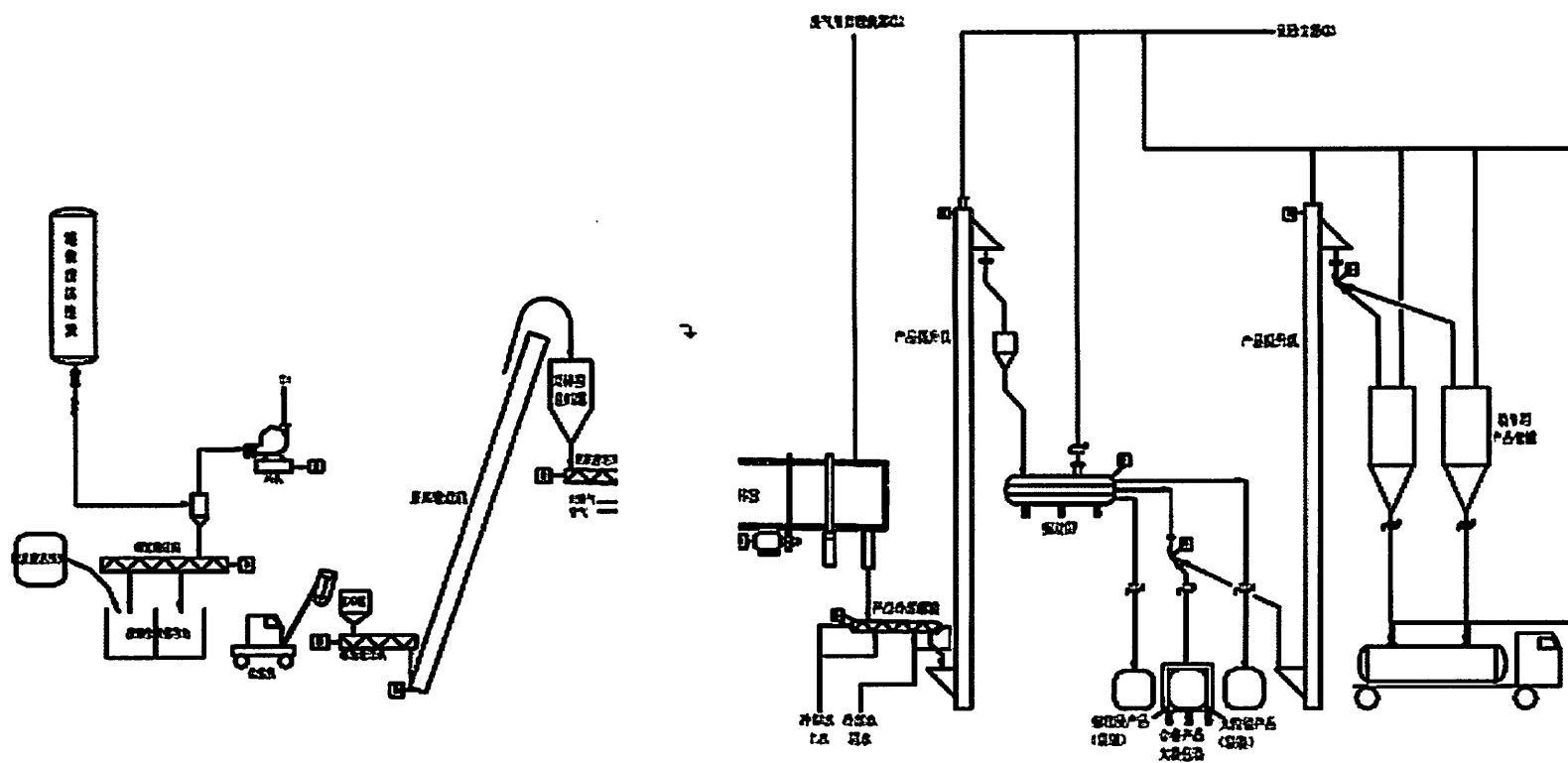
图 4.2-1 项目工艺流程图
