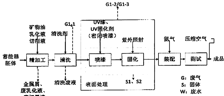
图 1 工艺流程图
